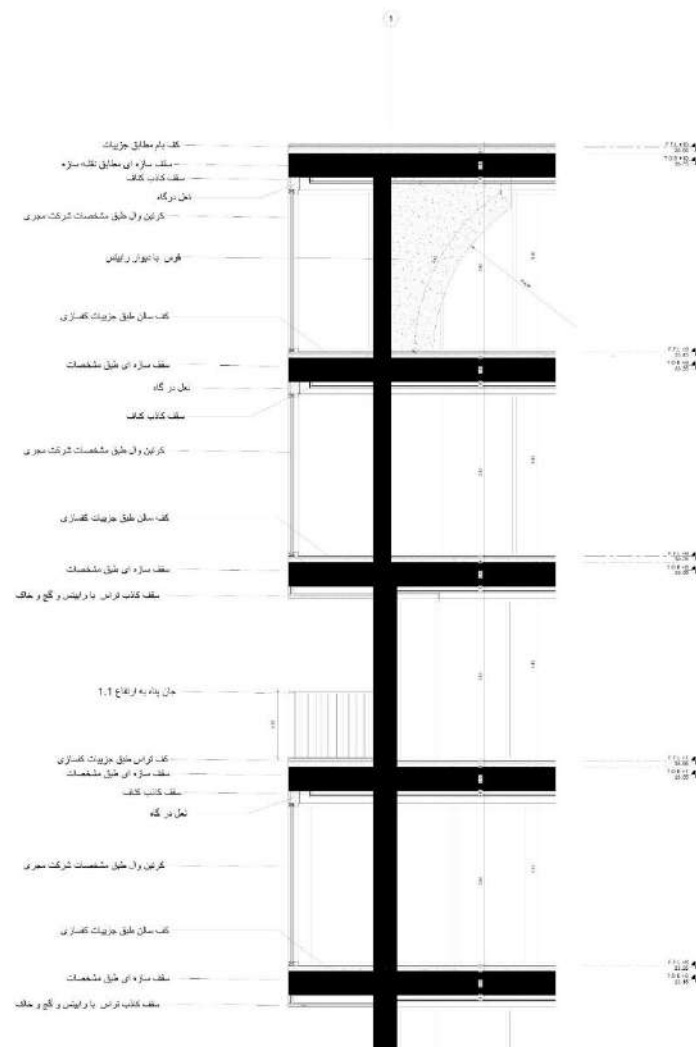
□ برش عمودی از جداره های خارجی با تاکید بر جزئیات اتصال عناصر نما به سازه اصلی با مقیاس ۱/۲۰ (wall section)
