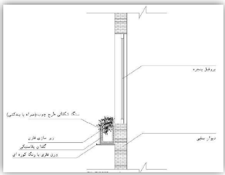
□ جزئیات عناصر الحاقی به نما
